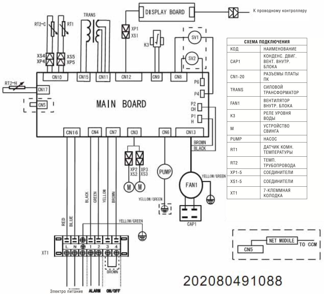
Рис. №4. Электрическая схема агрегатов ACF-60CM4, ACF-70CM4, ACF-105CM4.
