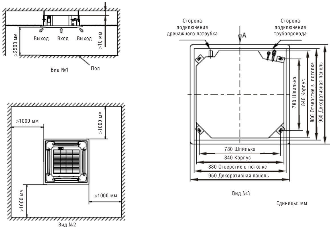
Рис. №6. Необходимое монтажное пространство для установки агрегатов.
