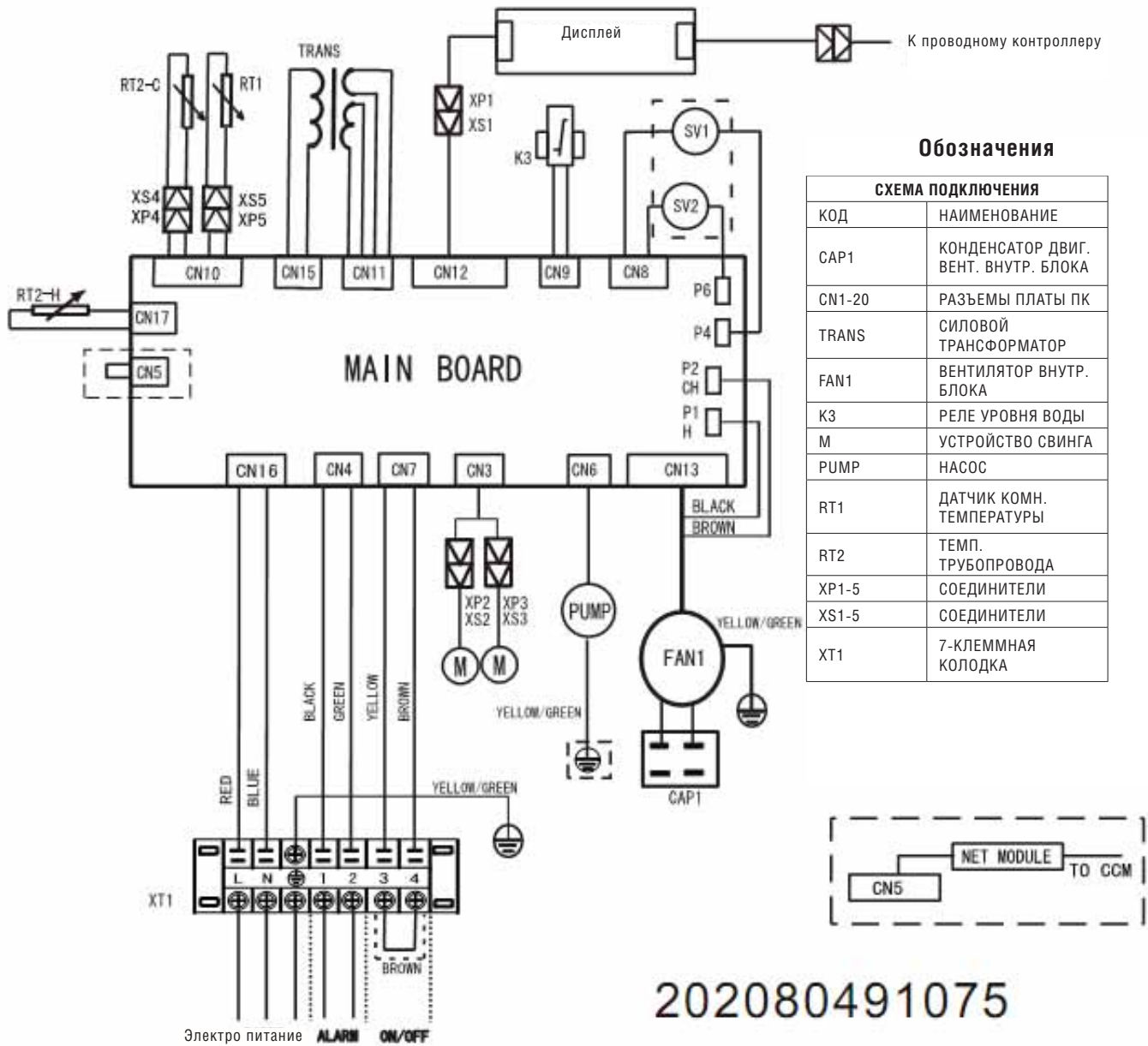
Рис. №3. Электрическая схема агрегатов АСF-50СМ4, АСF-65СМ4, АСF-95СМ4.
