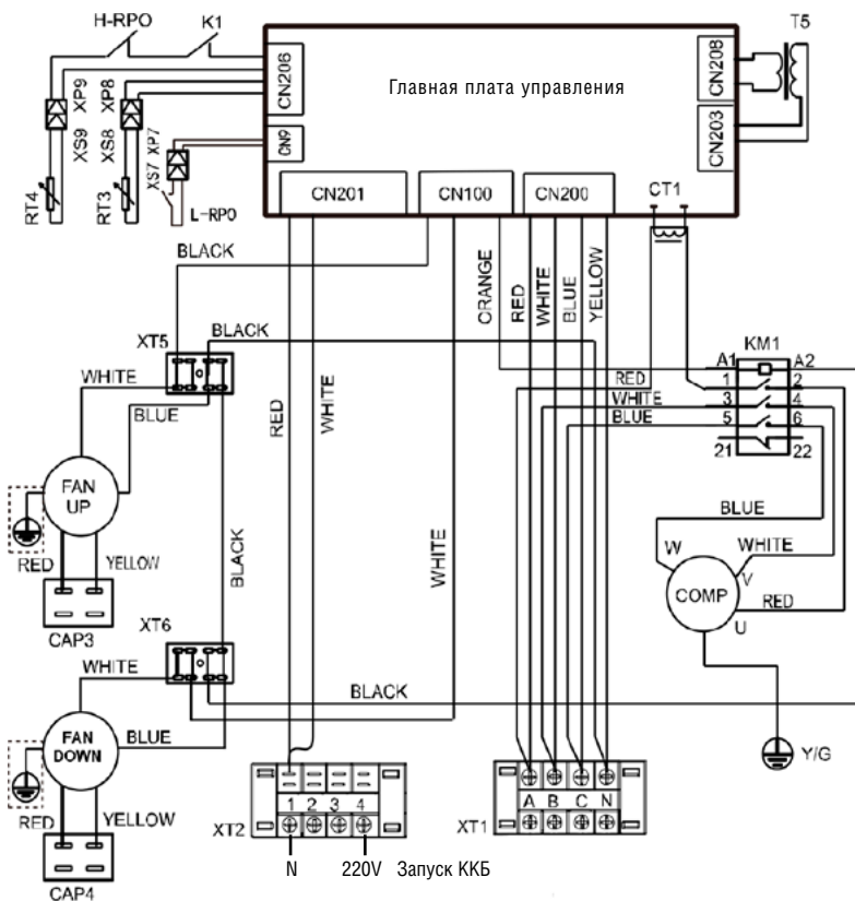
Рис.12. Электроподключение компрессорно-конденсаторных блоков АСQ-16/3
