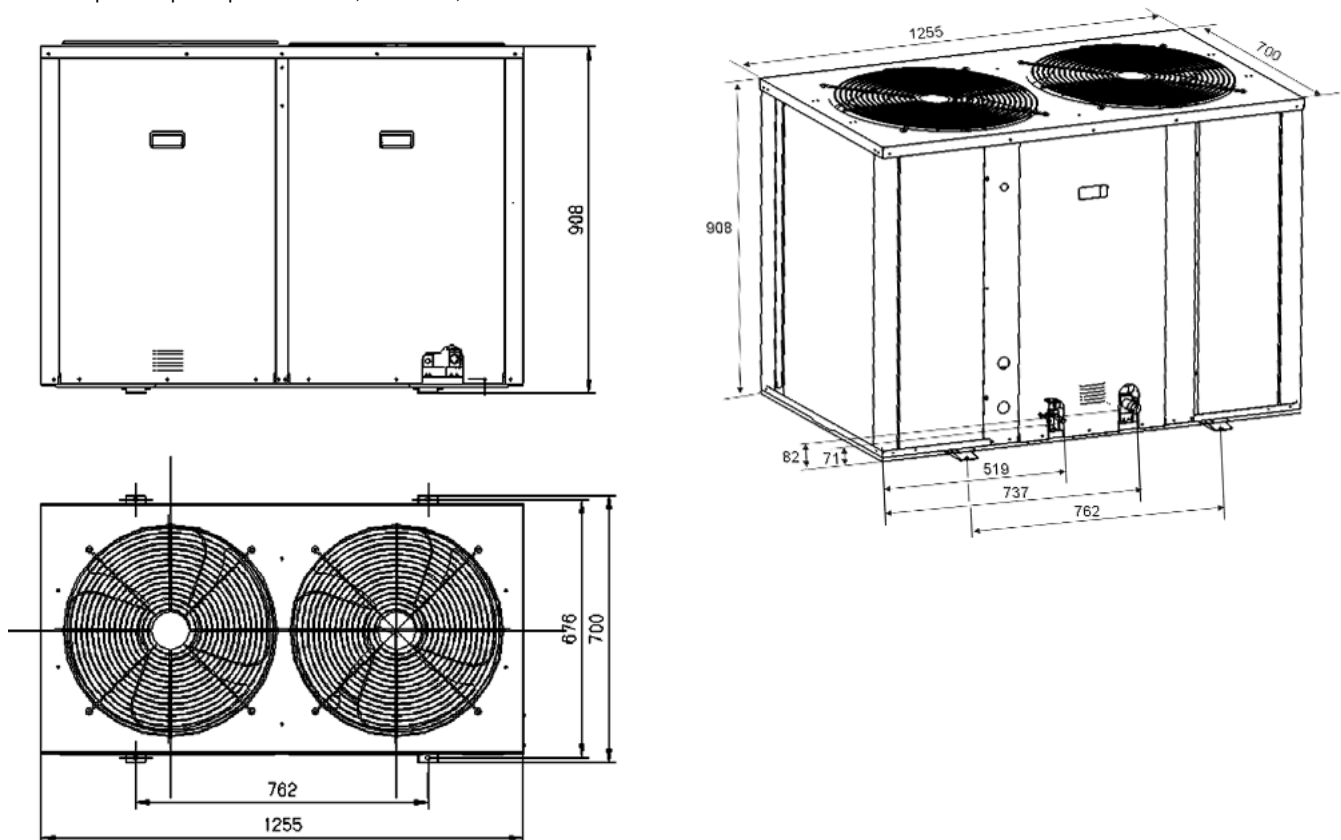
Рис. 4. Габаритные размеры АСQ-22/3, АСQ-28/3, АСQ-34/3
