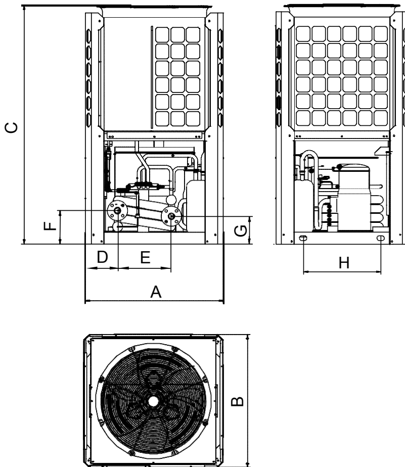
Модуль 25/35 кВт
