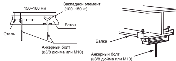
Рис. 4.2 Монтаж подвесов
