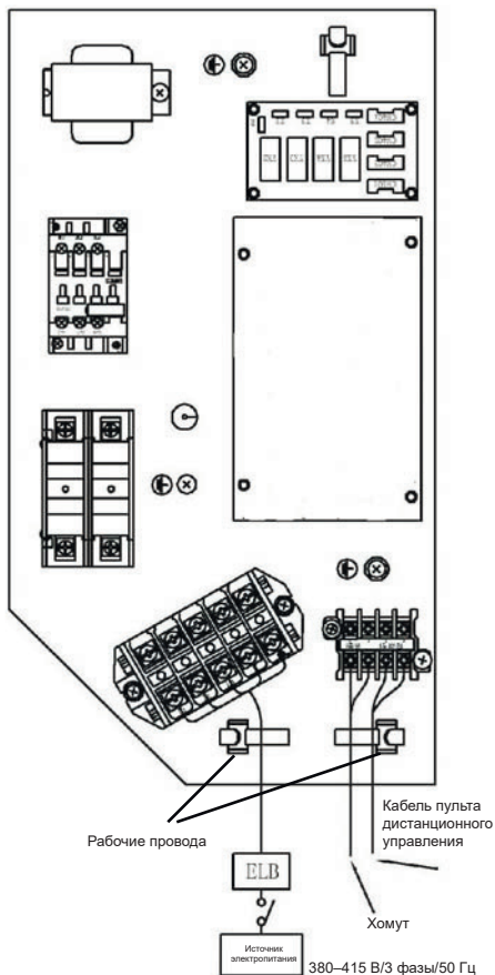
Рис. 7.2 Схема электрических подключений
