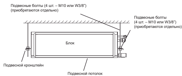
Рис. 4.4 Подвеска внутреннего блока
