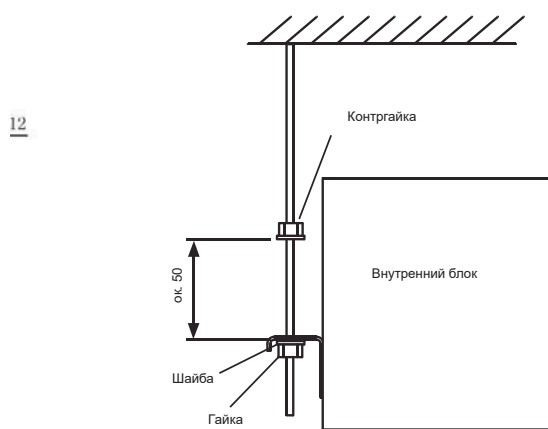
Рис. 4.5 Подвесные болты и гайки
