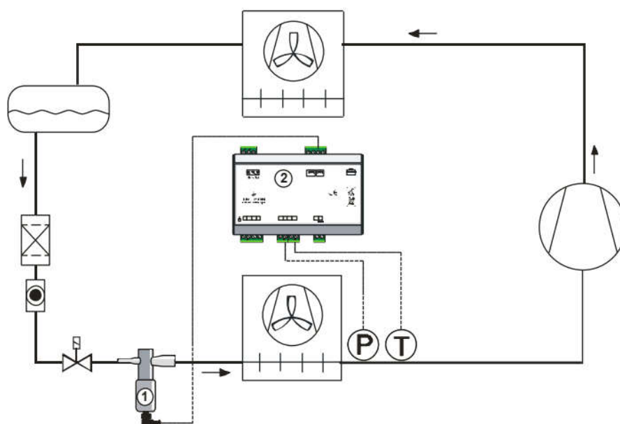
Рис.1 Расширительное устройство в холодильной системе
