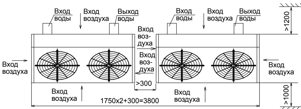
Рис. 2. Установка чиллера на фундамент
