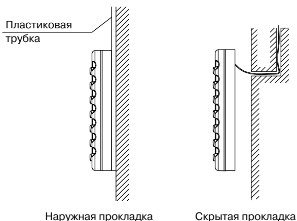
Рис. 3. Прокладка сигнального кабеля
