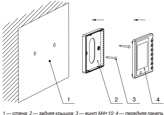
Рис. 4. Схема крепления проводного пульта
