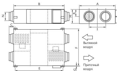
Модель RCS 1350-1500
